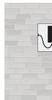
Cerrar la placa realizando una curva inferior con el cableado Connect the panel doing a lower curve with the wiring
